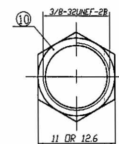
HEX NUT
