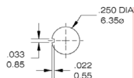
keyway
